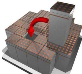
Рис. 2. Модульний принцип формування 256-елементної ЦАР
