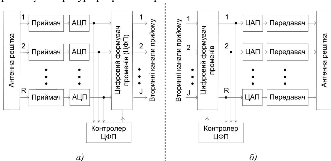
Рис. 1. Приймальний (а) та передавальний (б) сегменти ЦАР супутника-ретранслятора Thuraya
