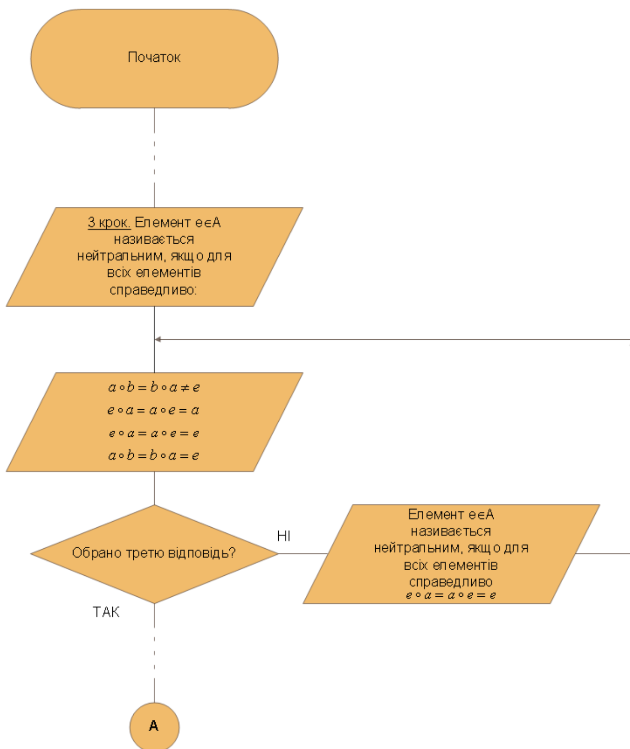
Рис. 4.1 – Блок-схема
